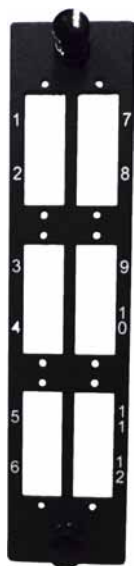
Placa Vertical
