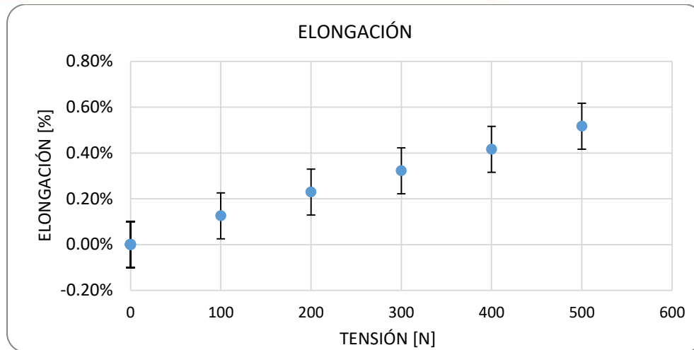
Figura 6. Elongación del cable bajo ensayo en función de la tensión aplicada
