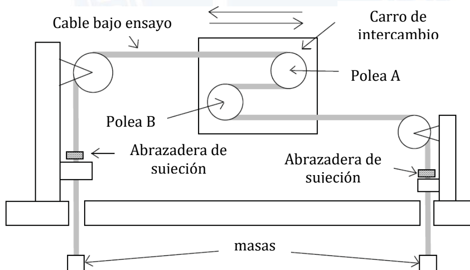
Figura 15. Diagrama esquemático del ensayo de flexión. Fuente IEC 60794-1-21-E8
