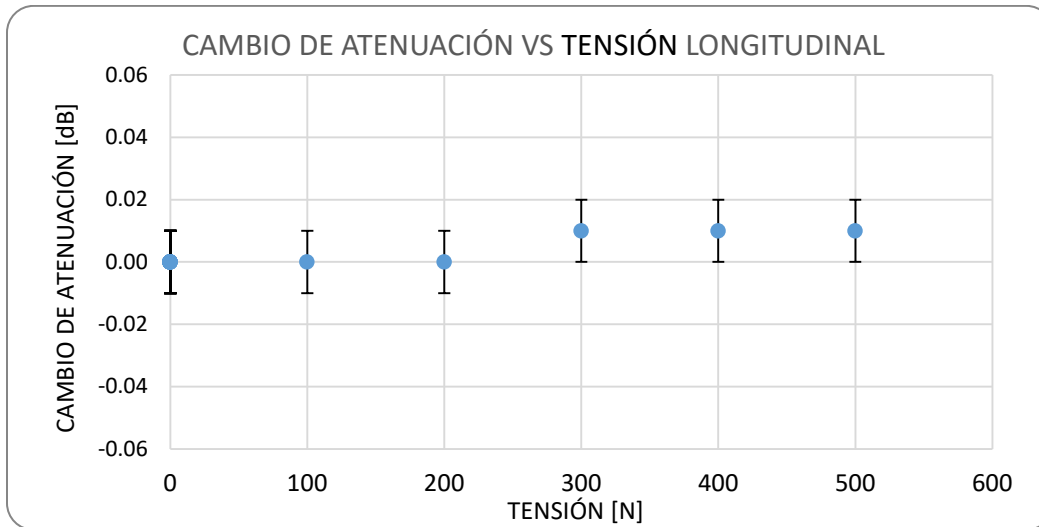
Figura 5. Cambio de atenuación del cable bajo ensayo en función de la tensión aplicada
