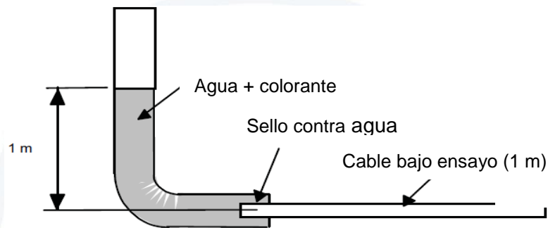
Figura 17. Diagrama esquemático del sistema de penetración de agua. Fuente IEC 60794-1-22-F5B
