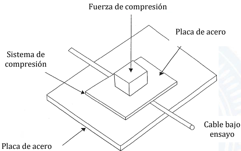
Figura 7. Diagrama esquemático del sistema de compresión. Fuente IEC 60794-1-21-E3
