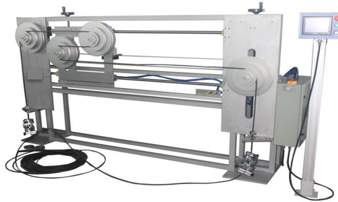
Figura 16. Máquina de flexión, norma internacional “IEC 60794-1-21 optical fiber cables – basic optical cable test procedures. Method 8 – Flexions”. Laboratorio de Pruebas Mecánicas, FIBERLAB S. DE R.L. DE C.V
