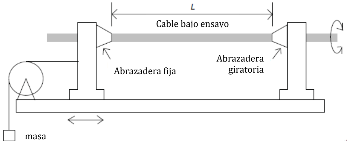
Figura 13. Diagrama esquemático del ensayo de torsión. Fuente IEC 60794-1-21-E7
