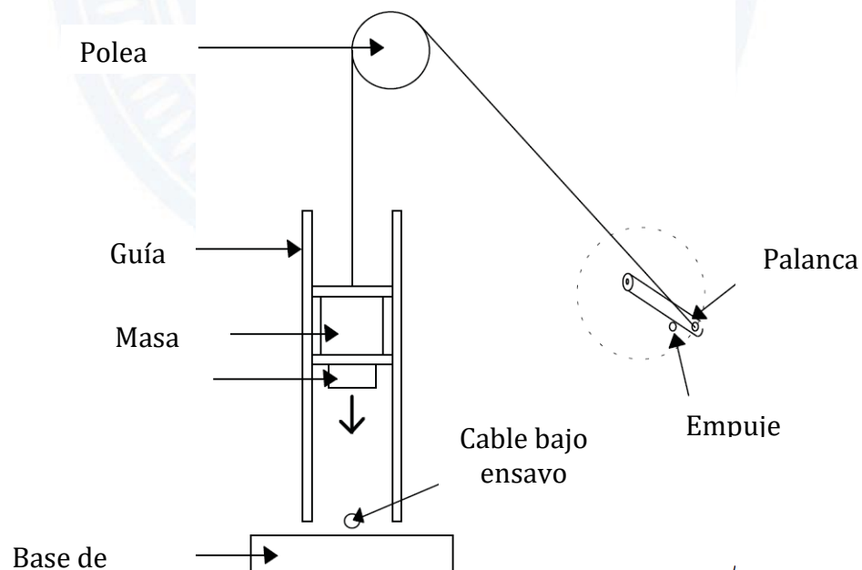
Figura 9. Diagrama esquemático del sistema de impacto. Fuente IEC 60794-1-21-E4
