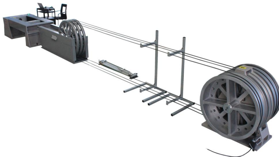
Figura 4. Máquina de tensión, norma internacional “IEC 60794-1-21 Optical fibre cables – Generic specifications -basic optical cable test procedures”. Method E1 – tensile performance” . Laboratorio de Pruebas Mecánicas. FIBERLAB S. DE R.L. DE C.V.
