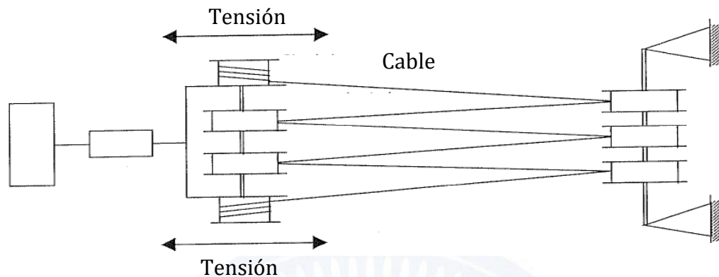
Figura 3: Diagrama esquemático del ensayo de tensión. Fuente IEC 60794-1-21-E1
