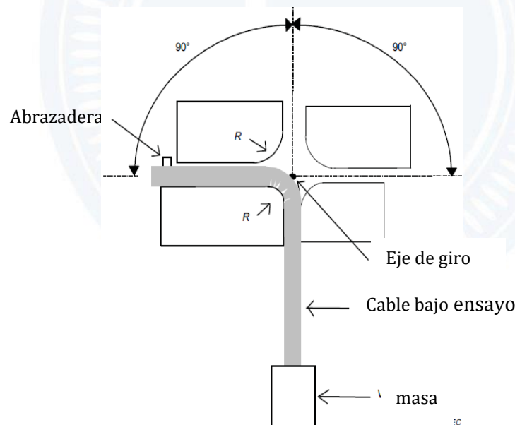
Figura 11. Diagrama del ensayo de dobleces repetidos. Fuente IEC 60794-1-21-E6
