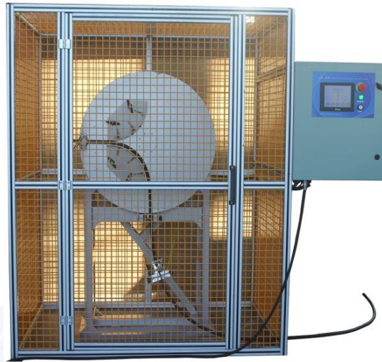
Figura 12. Máquina de dobleces repetidos, norma internacional “IEC 60794-1-21 optical fiber cables – basic optical cable test procedures. Method E6 – repeated bending”. Laboratorio de Pruebas Mecánicas. FIBERLAB S. DE R.L. DE C.V.
