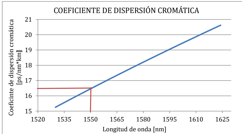
Figura 2. Coeficiente de dispersión cromática (CDC)
