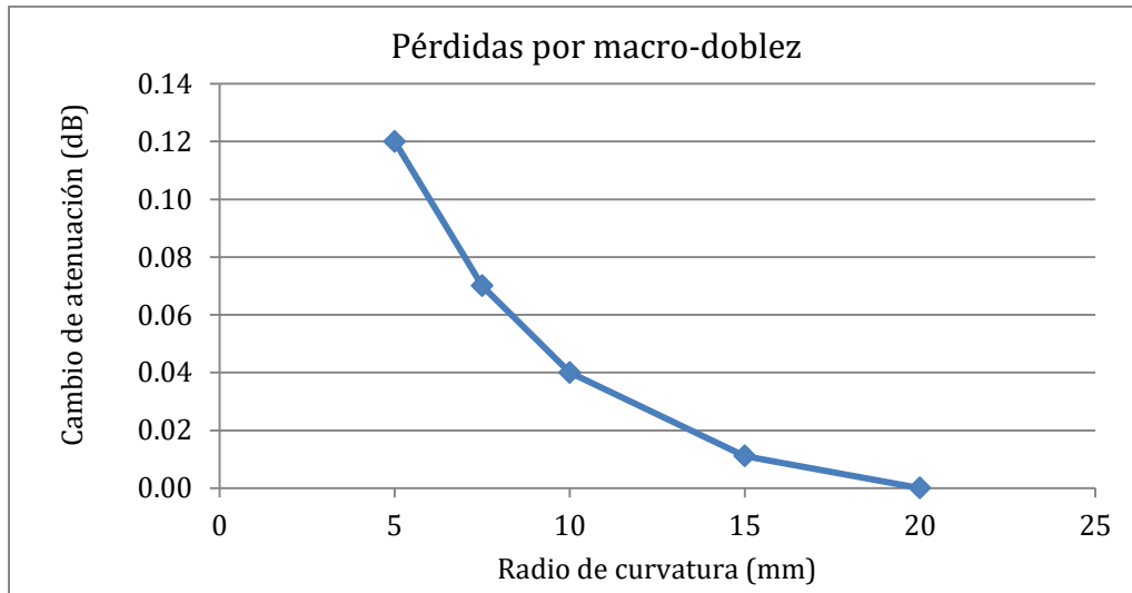
Figura 1. Curva de atenuación por macrocurvaturas
