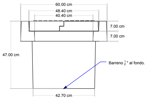
VISTA LATERAL REGISTRO
