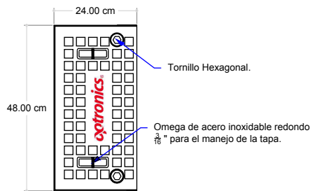
VISTA SUPERIOR TAPA "A" NOTA: LOGOTIPO EN COLOR ROJO
