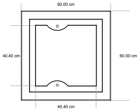
VISTA SUPERIOR REGISTRO
