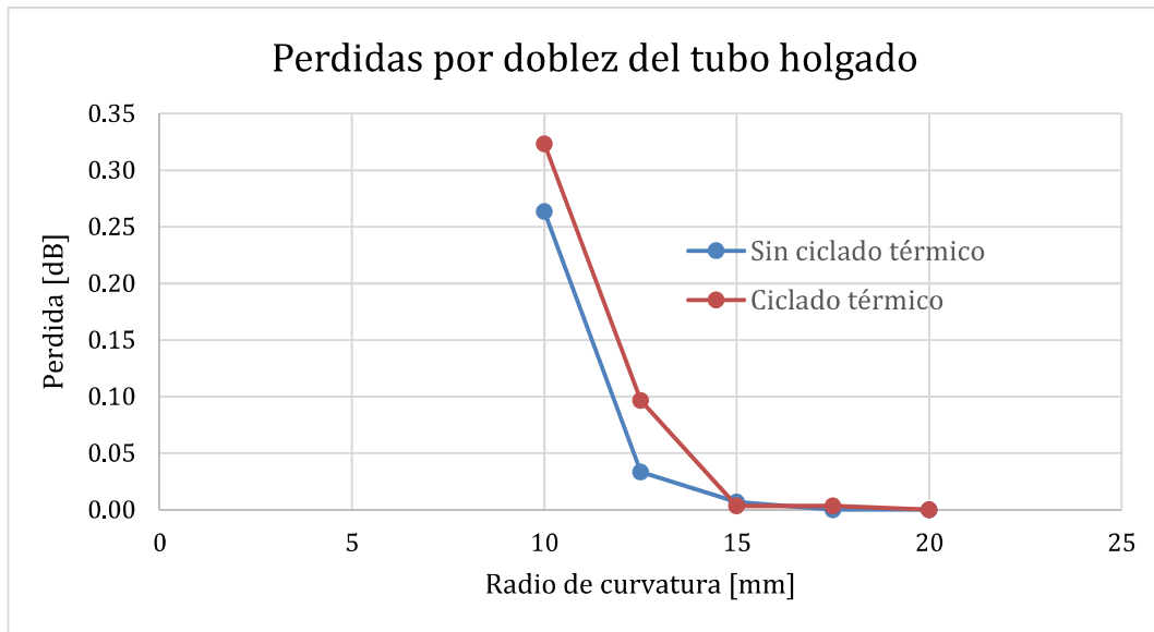
Figura 15. Curva de pérdidas por dobléz del tubo holgado a 1550 nm
