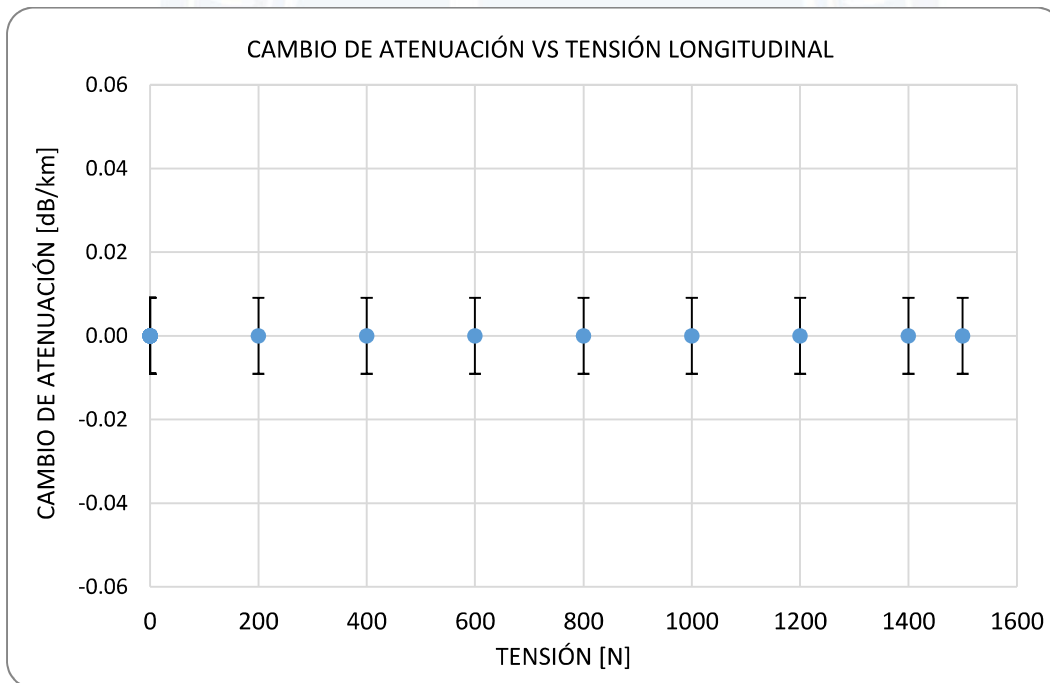
Figura 3. Cambio de atenuación del cable bajo ensayo en función de la tensión aplicada
