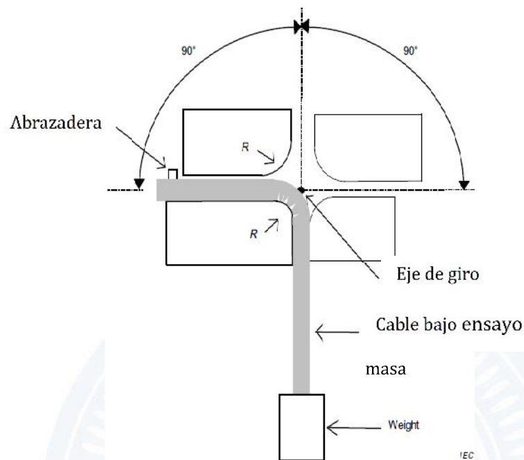
Figura 9. Diagrama del ensayo de dobleces repetidos. Fuente IEC 60794-1-21-E6
