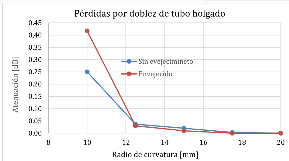
Figura 15. Curva de pérdidas por doblado del tubo holgado a 1550 nm
