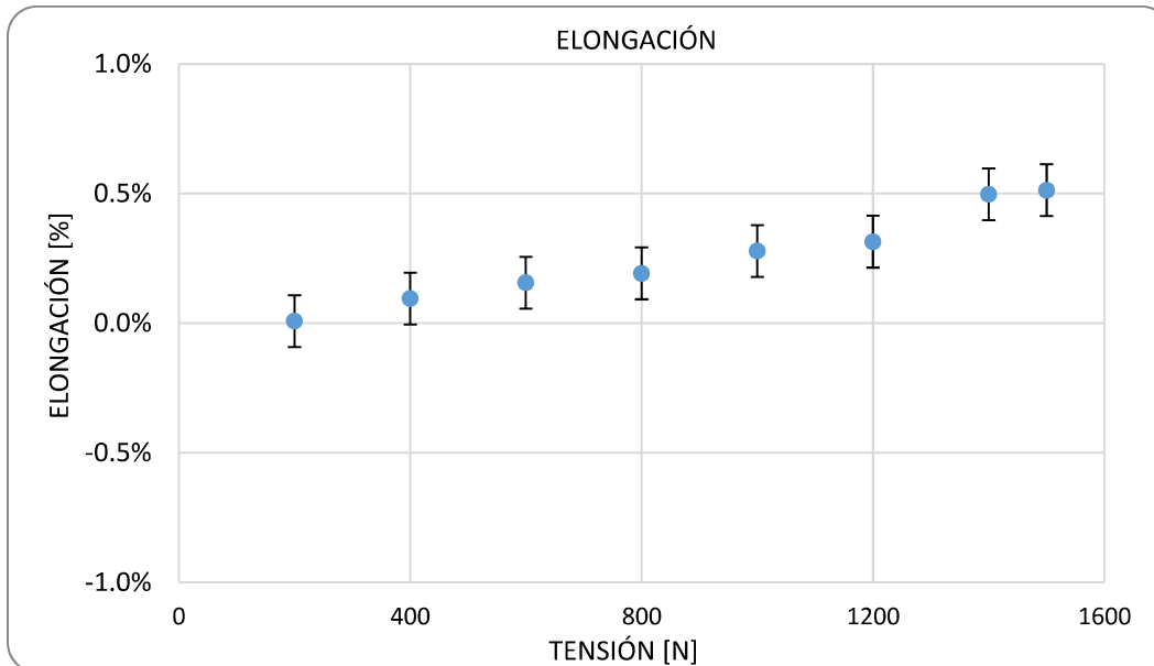
Figura 4. Elongación del cable bajo ensayo en función de la tensión aplicada
